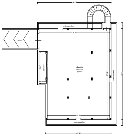
PIANTA PIANO INTERRATO ESISTENTE Permesso di Costruire n°228 del 23.07.2010
