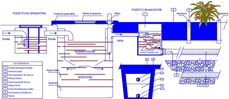
SEZIONE - Vasca Imhoff e Impianto di Dispersione
