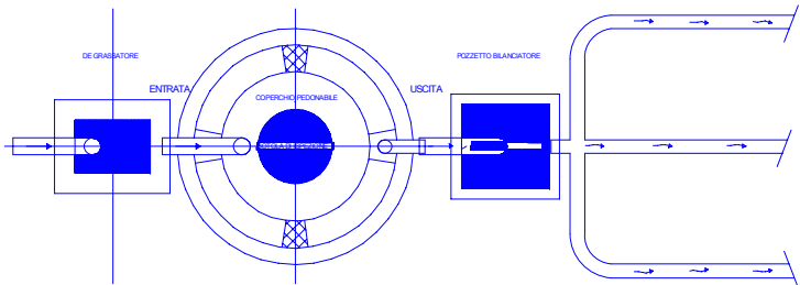
PIANTA - Vasca Imhoff e Impianto di dispersione
