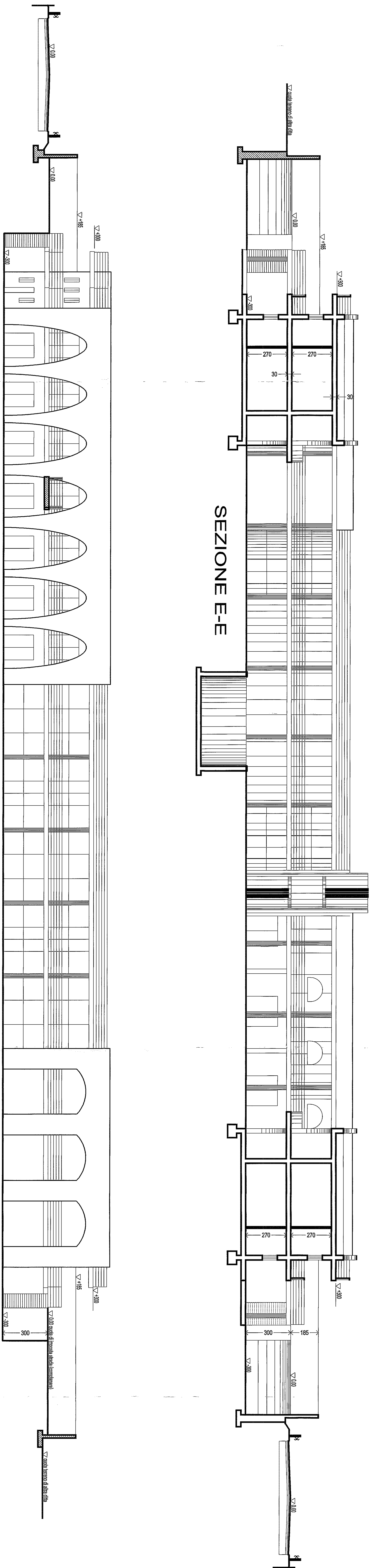
SEZIONE D-D
