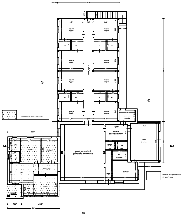
PIANTA PIANO TERRA AMPLIATA DA REALIZZARE
