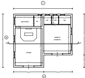
PIANTA PIANO TERRA DA REALIZZARE
