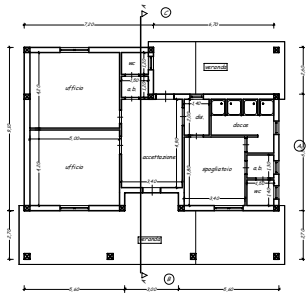
PIANTA PIANO TERRA ESISTENTE DA MODIFICARE AD UFFICI
