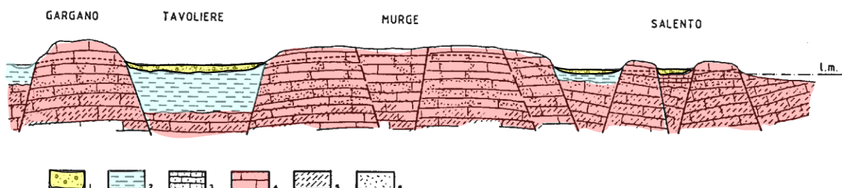
Fig. 2 : Sezione idrogeologica schematica della Puglia in direzione NO-SE. 1. Depositi alluvionali (Olocene-Pleistocene sup.); 2. Argille grigio azzurre (Pleistocene inf.-Pliocene); 3. Calcareni mioceniche; 4. Calcari di piattaforma apula (Cretaceo); 5. Sup.piezometrica H 2 O salata; 6. Sup.piezometrica H 2 O dolce.
