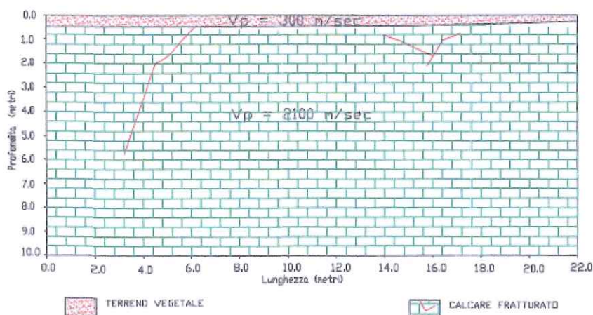
profilo stratigrafico ottenuto 1
