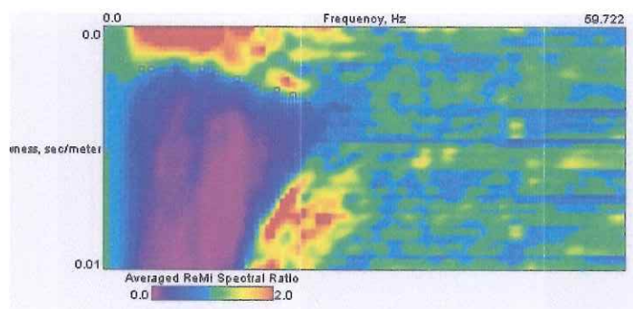
Fig. 2 Esempio di picking
